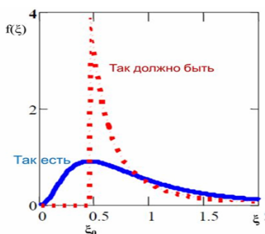
Рис. 3: Распределения Туганова-Цзя и Парето
