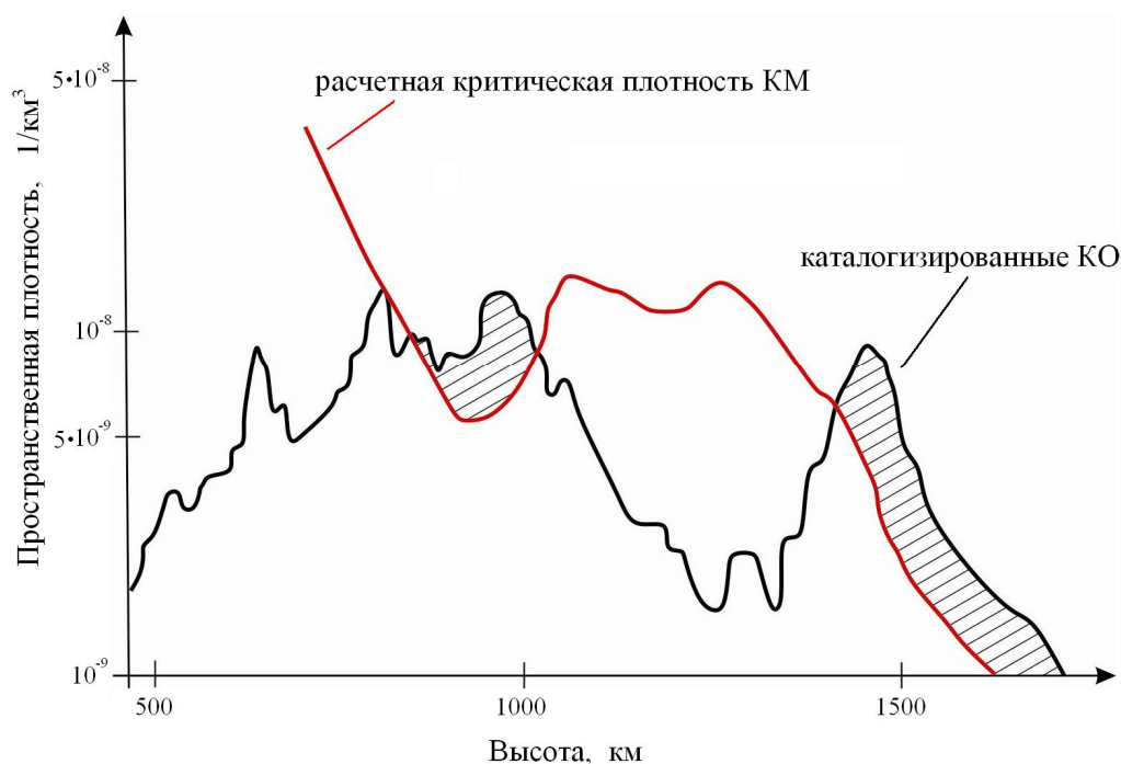
Рисунок 4. Критическая плотность в области низких орбит
