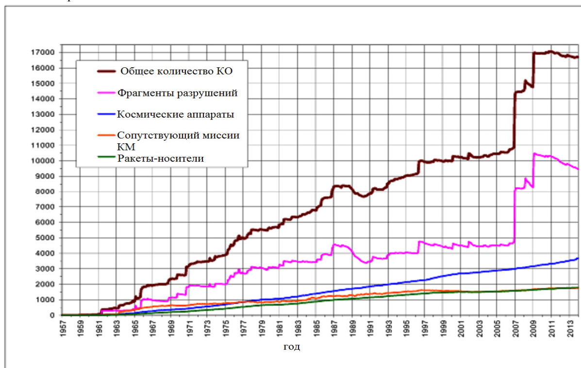
Рисунок 1. Рост техногенной засоренности ОКП за весь период освоения космоса
